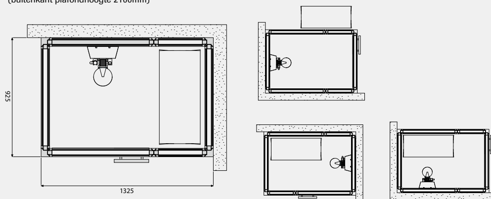
Tylö stoomdouche i130 (buitenkant plafondhoogte 2100mm)
