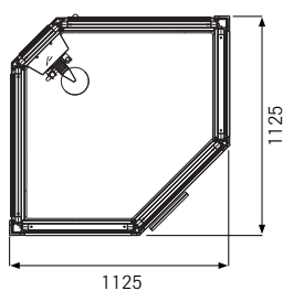
Tylö stoomdouche i110/c (Art. no. 9607 4630)
