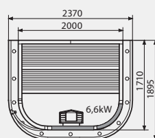
Midi Vision (Externe dakhoogte 2030 mm)
