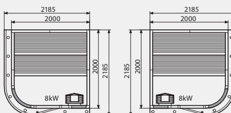
Midi Vision (Externe dakhoogte 2030 mm)
