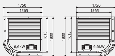
Space Vision 150, hoek instap (Externe dakhoogte 2030 mm)
