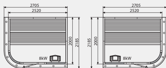
Space Vision 250, front instap (Externe dakhoogte 2030 mm)
